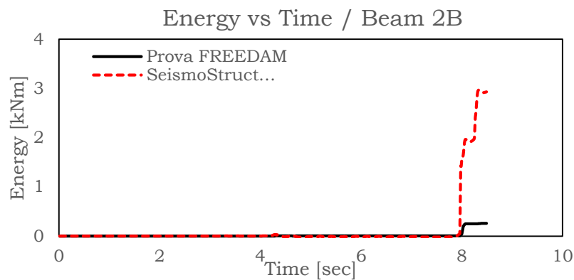
Fig. 5.223 - Energy vs time - Bema 2B - FREEDAM
