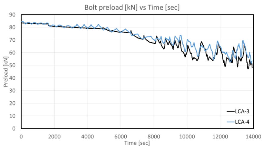
Fig. 4.49 – Bolt preload vs Time - Right side
