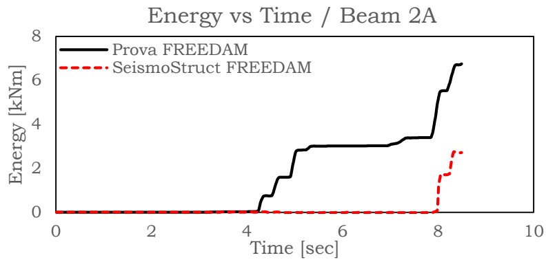
Fig. 5.221 - Energy vs time - Bema 2A - FREEDAM
