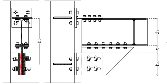
Fig. 4.3 – Lever arm of friction joints: a) configuration n.1; b) configuration n.2
