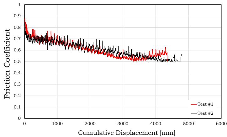
Fig. 2.12 – Actual friction coefficient – M4
