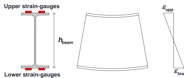
Fig. 5.192 – Curvature
