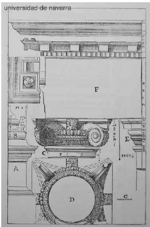
Figura 56 – Capitel jônico, Scamozzi. Fonte: http://www.unav.es/ha/003-ORDE/partes-capiteles-jonico.htm
