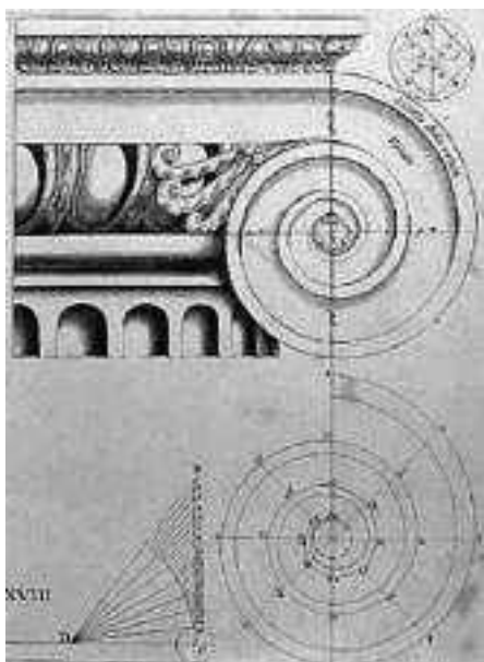
Figura 59 – Detalhe de capitel jônico, Vignola. Fonte: http://www.unav.es/ha/009-TRAT/vignola-regole.htm
