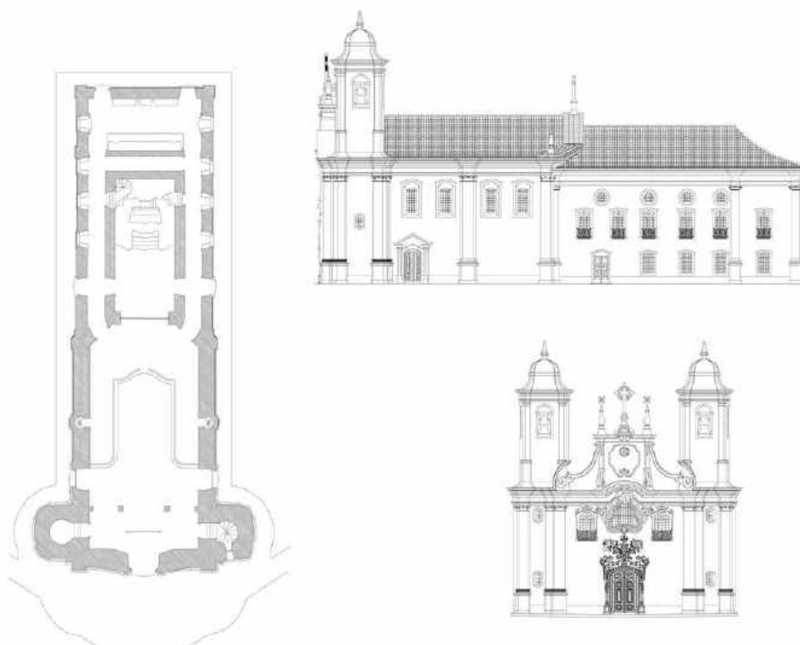
Figura 1 – Planta, elevação e frontispício da Capela do Carmo. Fonte: DANGELO, André. A cultura arquitetônica em Minas Gerais...
