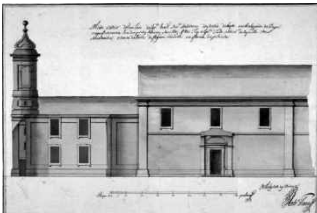
Figura 62 – “Alçado Exterior de um lado da Igr.ª de N. Sr.ª do Socorro do Sertão de Baía no qual se mostra hua das portaz travessas, janellaz q dão Luz à Igr.ª, Lado Exterior da Capella Mor, Sanchrestia, evista da Torre de Figura Redonda na forma da planta”. Risco do Arquitecto das Ordens Militares, Rodrigo Franco. Fonte: ANTT, PT-TT-MR/1/9
