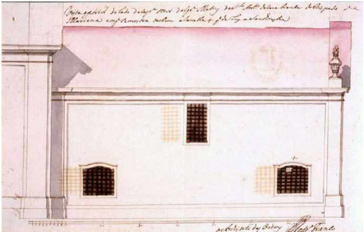
Figura 18 – “Vista exterior do lado da Cap.ª Mor da Igr.ª Matriz de St.º Ant.º da Casa Branca do Bispado de Mariana em qse mostra taobem a Janella + qda Luz a Sanchrestia”. Rodrigo Franco. Fonte: ANTT-PT-TT-MR/1/14
