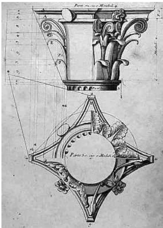
Figura 40 – Capitel coríntio, Vignola. Regla de las cinco ordenes de Jacome de Vignola . Fonte: < http://www.unav.es/ha/009-TRAT/vignola-regole.htm >
