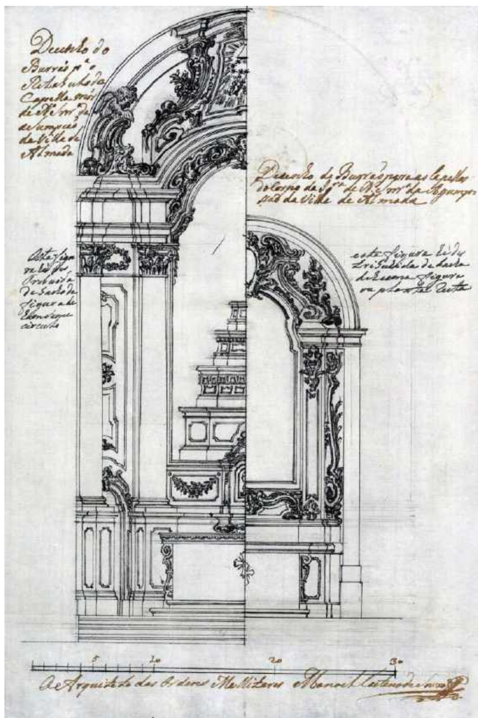
Figura 73 – “Desenho do Borrão p. a Retábulo da Capela Mór de N. Sra. a da Assumpção da Vila de Almada”, pelo “Arquiteto da Ordens Militares” Manoel Caetano de Souza. Fonte: ANTT: PT-TT-MR/1/19
