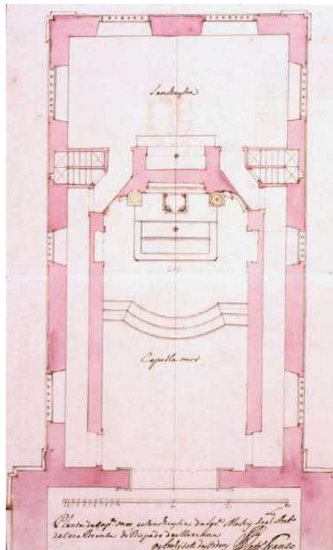
Figura 13 – “Planta da Cap. a mor, e sanchresia da Igr. a Matriz de St. o Antonio da Casa Branca do Bispado de Mariana. O Archyteto das Ordens Rodr. o Franco”. Fonte: ANTT-PT-TT-MR/1/15.
