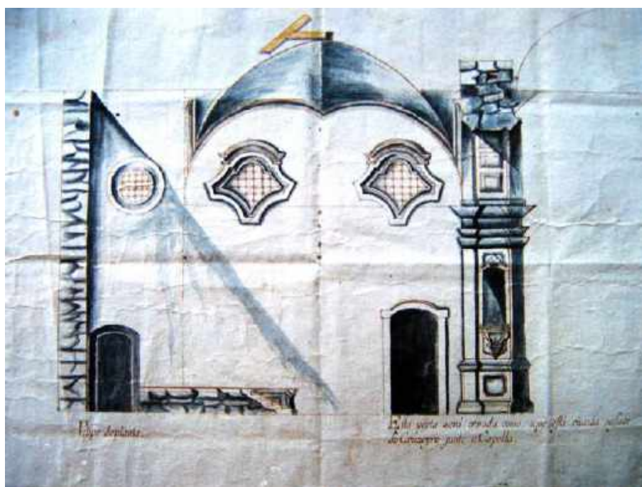
Figura 101 – Risco em elevação da capela-mor de São Francisco de Assis, atribuído ao Aleijadinho. Museu da Inconfidência , Ouro Preto, com destaque para delineamento da abóbada do forro em dois tramos
