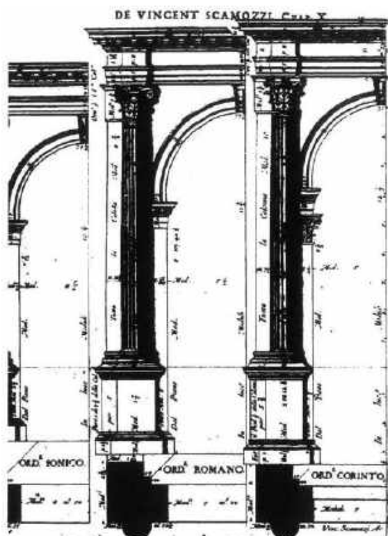
Figura 44 – Ao centro, Ordem ou Gênero “Romano” de Scamozzi. Fonte: < http://www.unav.es/ha/009-TRAT/scamozzi.htm >.
