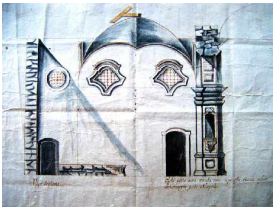
Figura 8 – Risco em elevação da capela-mor da Capela de São Francisco, atribuído ao Aleijadinho. Destaque para iluminação zenital e sombreamento. Museu da Inconfidência , Ouro Preto
