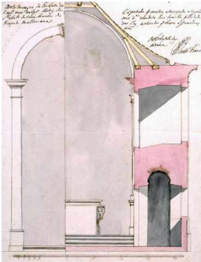
Figura 14 – “Espaçado q’ mostra atravessada a Capella mor d. a vendose huá janela qlhehade dar Luz, e ecorredor q busca a sanchrestia”. Rodrigo Franco. Fonte: ANTT- PT-TT-MR/1/16
