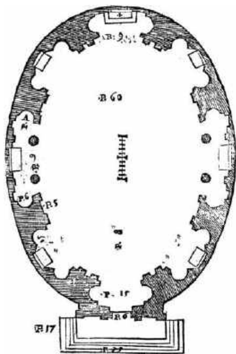
Figura 12 – Planta oval no Livro Quinto de Arquitetura, Delli Tempii , de Sebastiano Serlio, fl. 204v. Fonte: < http://gallica.bnf.fr/ >.
