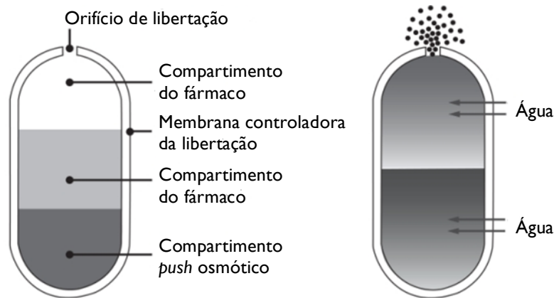
Figura I – Sistema OROS Push-Pull multicamada.
