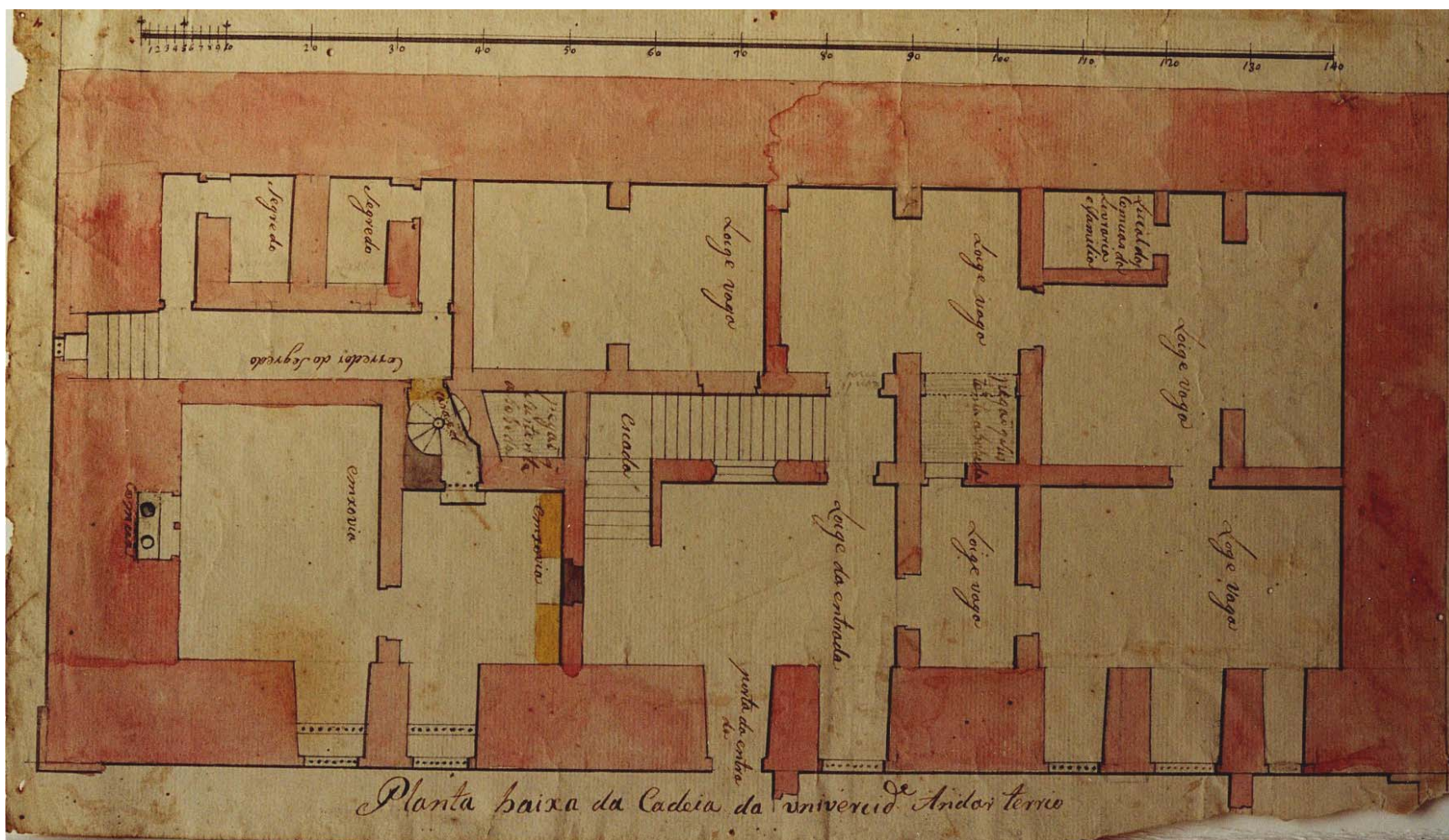
Planta da cadeia universitária (José do Couto, 1819, MNMC).
