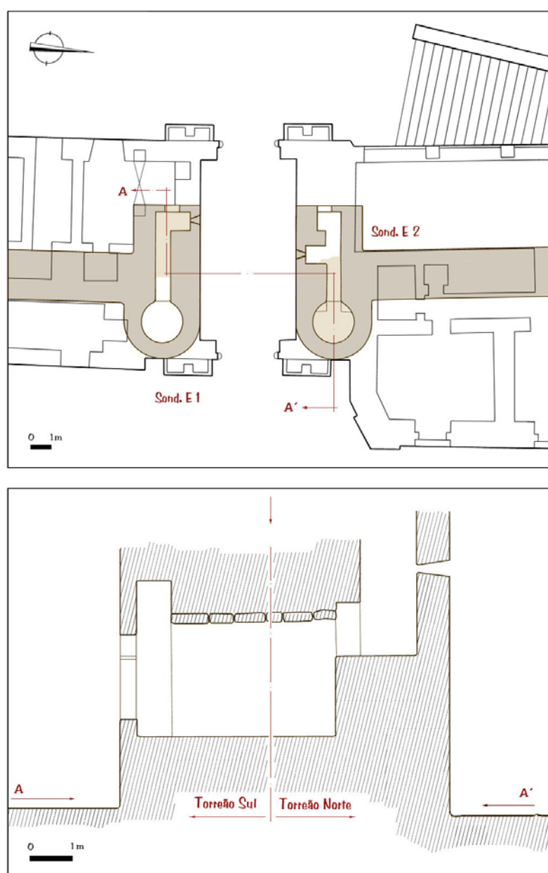
Planta e corte das Sondagens E1 e E2 (des. José Luís Madeira).
