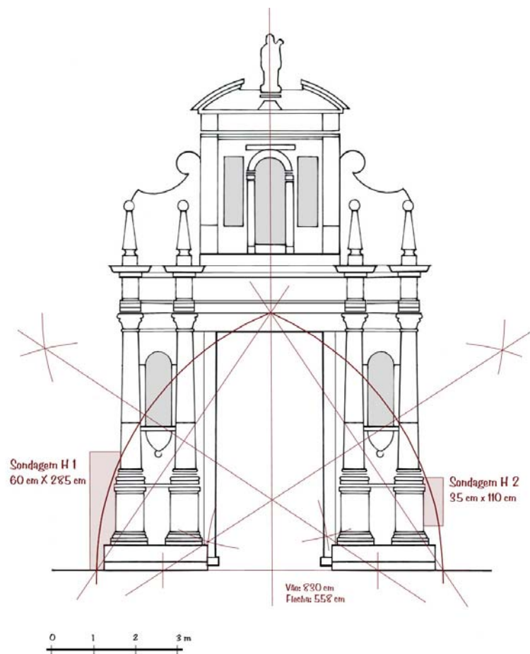
Alçado das Sondagens H1 e H2 (José Luís Madeira).
