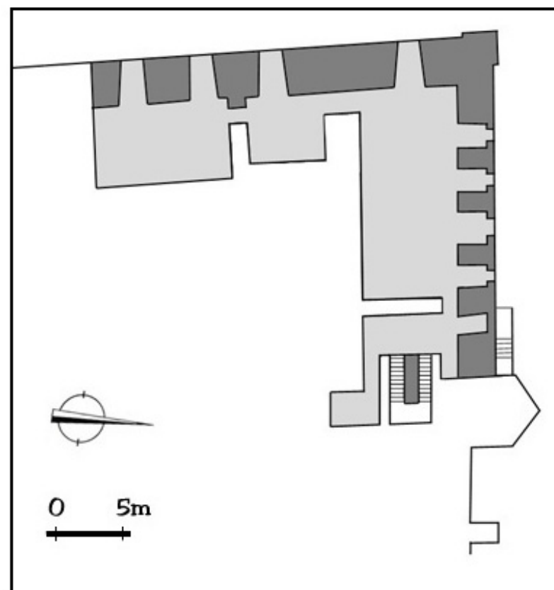
Planta das infra-estruturas do ângulo NO dos Gerais com a(s) sala(s) ocupada(s) pelo Arquivo da Universidade (José Luís Madeira).
