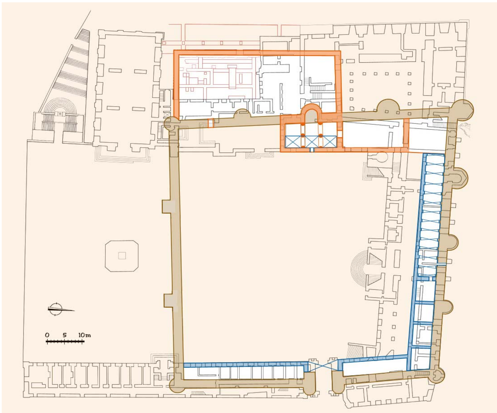
Implantação do Paço Real da Alcáçova ao tempo de D. Afonso IV (des. José Luís Madeira).
