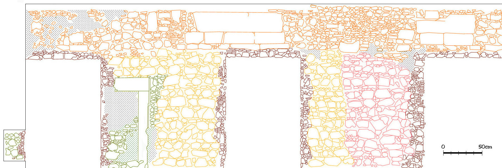
Alçado da Sondagem G1 (des. José Luís Madeira).
