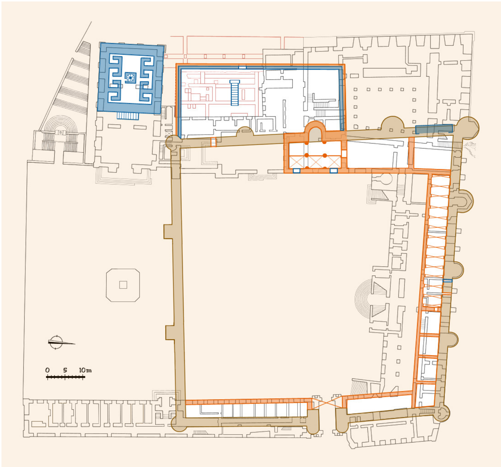
Implantação das intervenções realizadas por D. João I no Paço Real da Alcáçova (des. José Luís Madeira).
