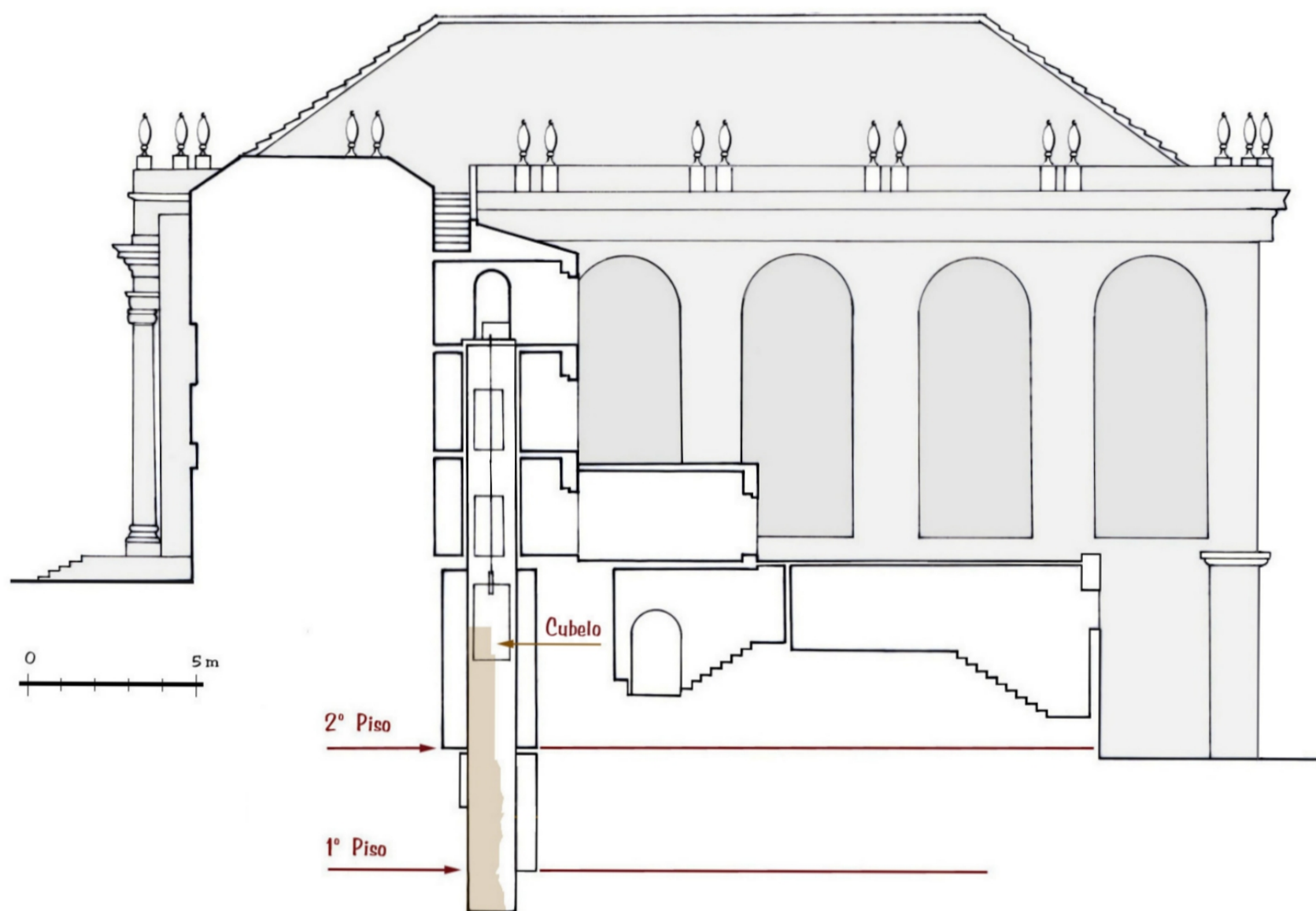
Corte transversal das estruturas e caixa do elevador da Biblioteca Joanina (des. José Luís Madeira).
