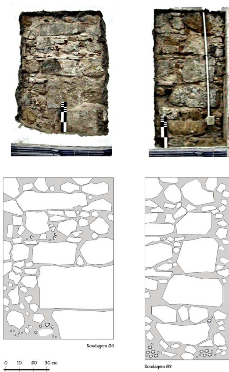
Aspectos e alçados das Sondagens G3 e G4 (José Luís Madeira).
