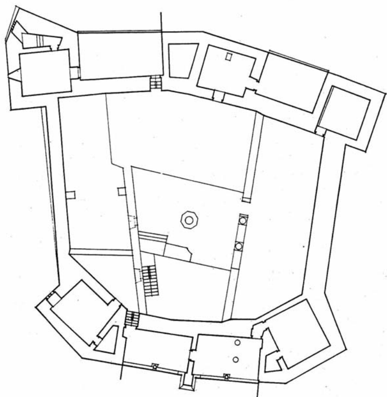
Planta do Castelo de Porto de Mós.
