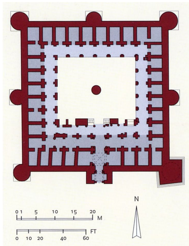
Planta do ribat de Susa (Magreb).
