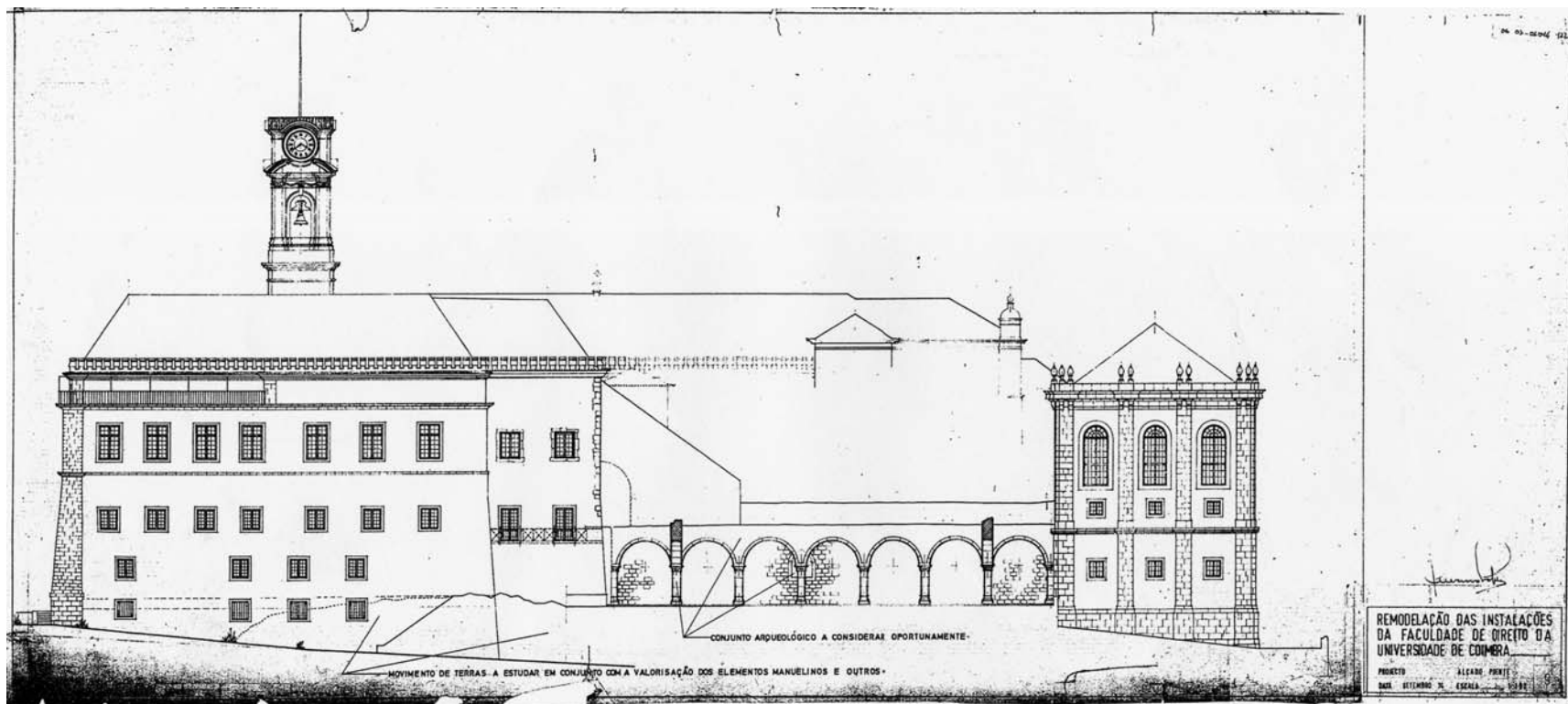
Alçado poente do Paço das Escolas com a marcação dos movimentos de terras projectados na década de 1960 (DGEMN).
