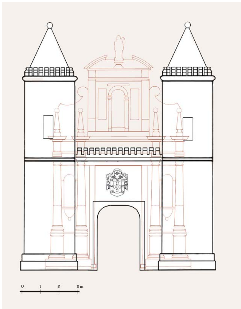
Hipótese de reconstituição do alçado externo da porta-forte manuelina (des. José Luís Madeira).
