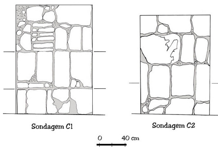
Alçado das Sondagens C1 e C2 (des. José Luís Madeira)
