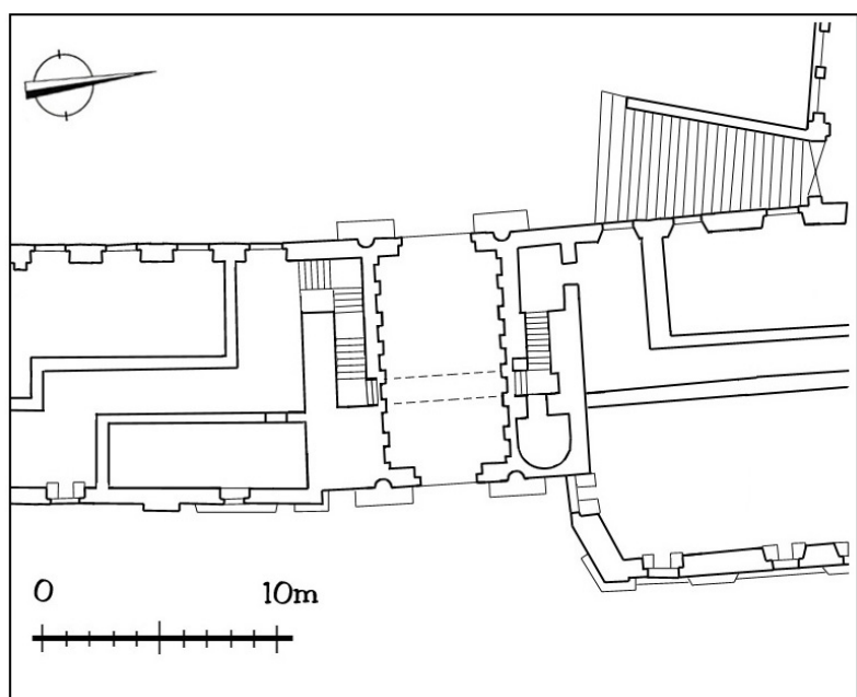
Planta da Porta Férrea ao nível do 1º piso.
