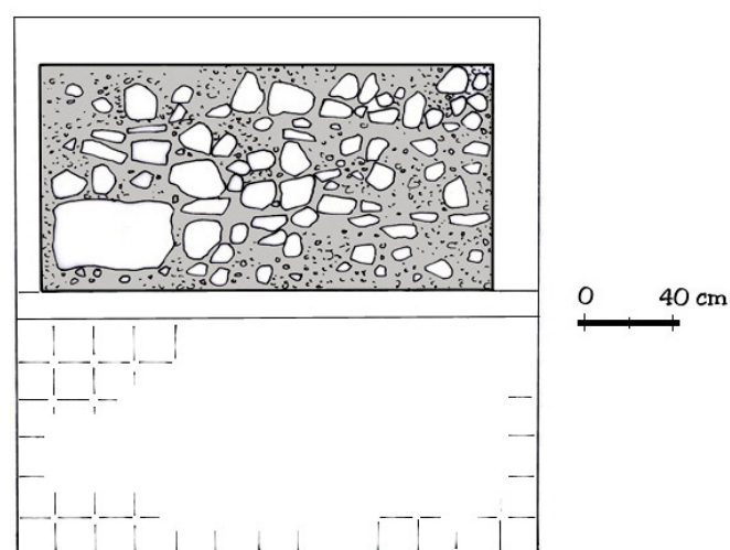
Aspecto e alçado da Sondagem D3 (des. José Luís Madeira).
