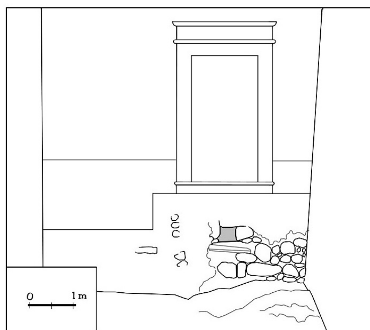
Cloaca da fachada norte: aspecto e alçado (José Luís Madeira).
