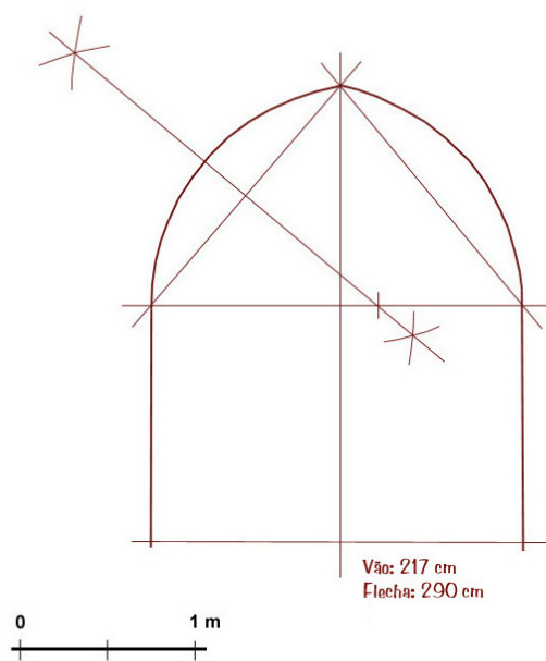
Reconstituição do traçado da porta de arco quebrado (José Luís Madeira).
