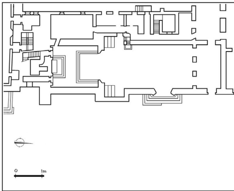
Planta da Capela de S. Miguel (José Luís Madeira).
