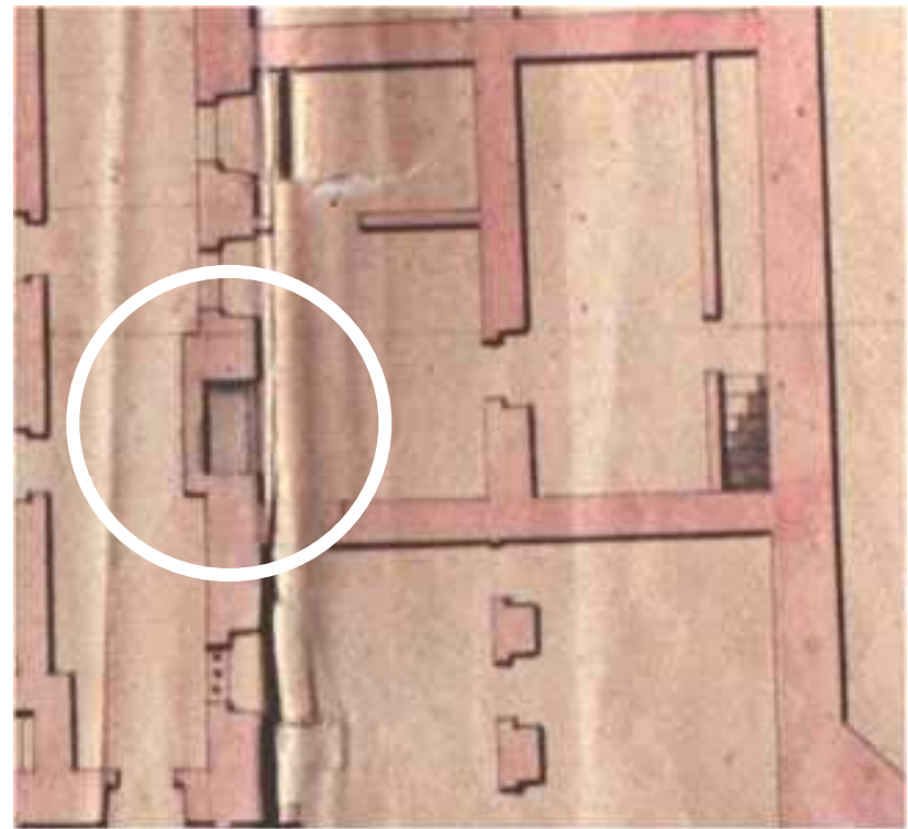
Pormenor da planta pombalina ilustrando a lareira das câmaras do bispo.
