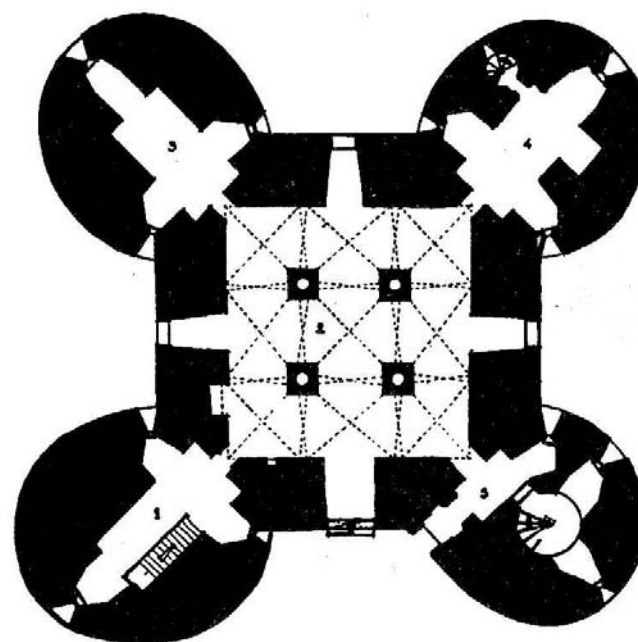
Planta do Castelo de Évora-Monte.
