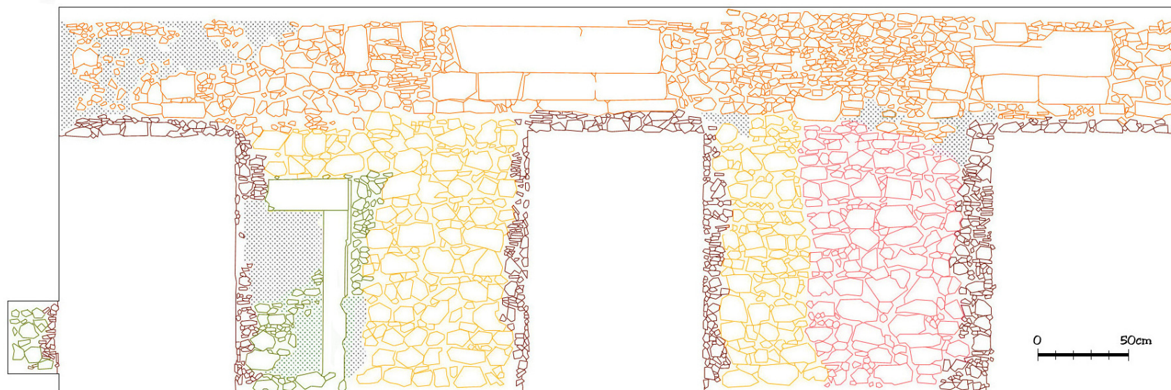
Alçado da Sondagem G1.
