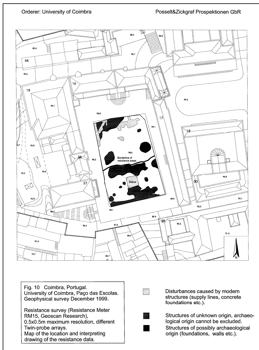
Resultado da prospecção geofísica no Pátio da Universidade.
