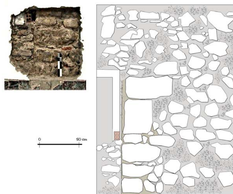
Aspecto e alçado da Sondagem G5 (José Luís Madeira).
