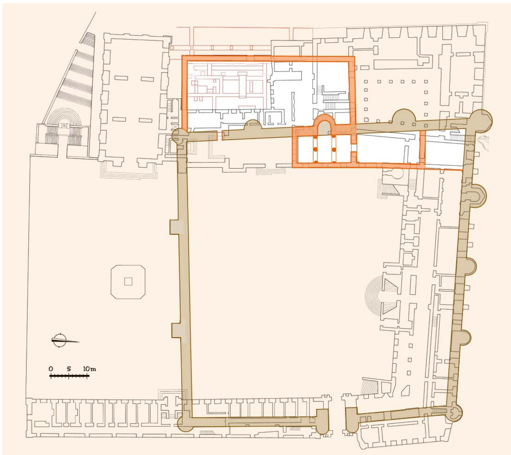
Implantação do albacar e da capela e aula do palatium primitivo (José Luís Madeira).
