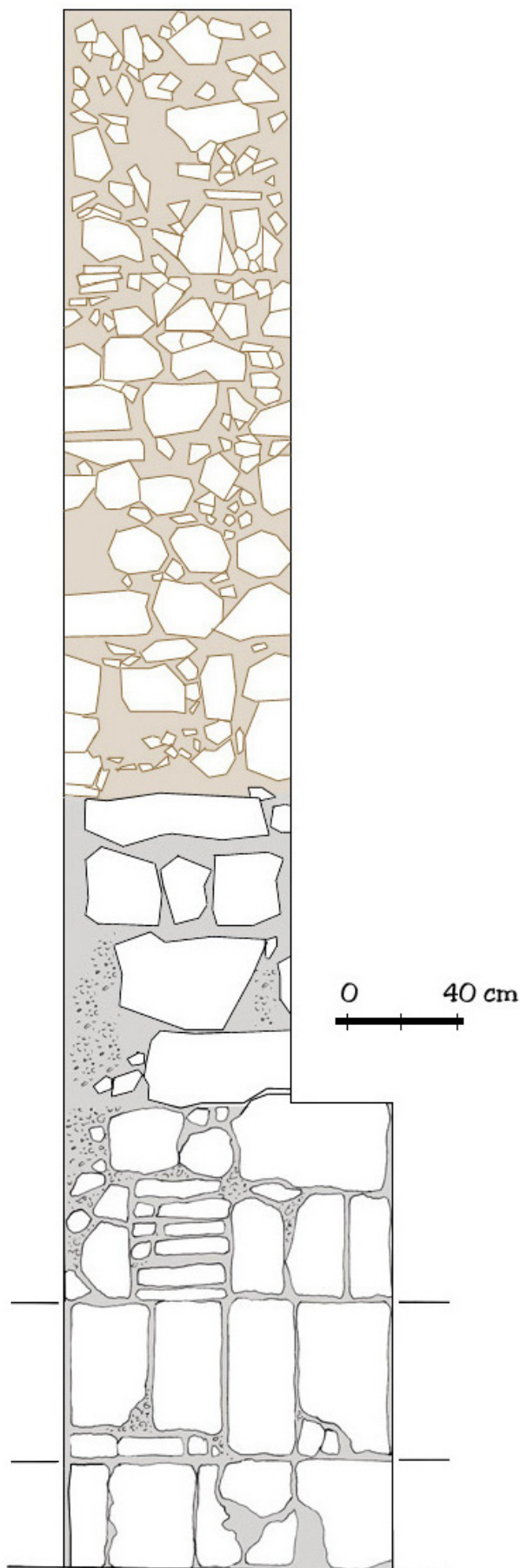
Alçado da sondagem realizada no torreão angular nordeste (des. José Luís Madeira).
