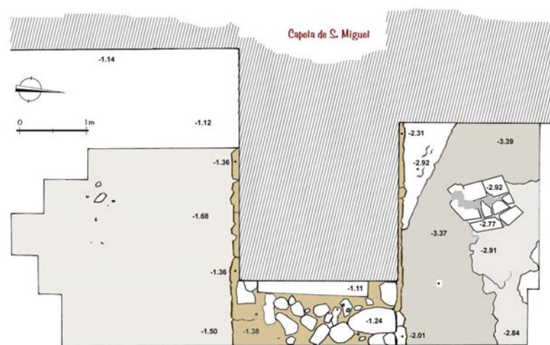
Planta da Sondagem A2 . Campanha arqueológica de Jun./Ag. 2000 (des. José Luís Madeira).
