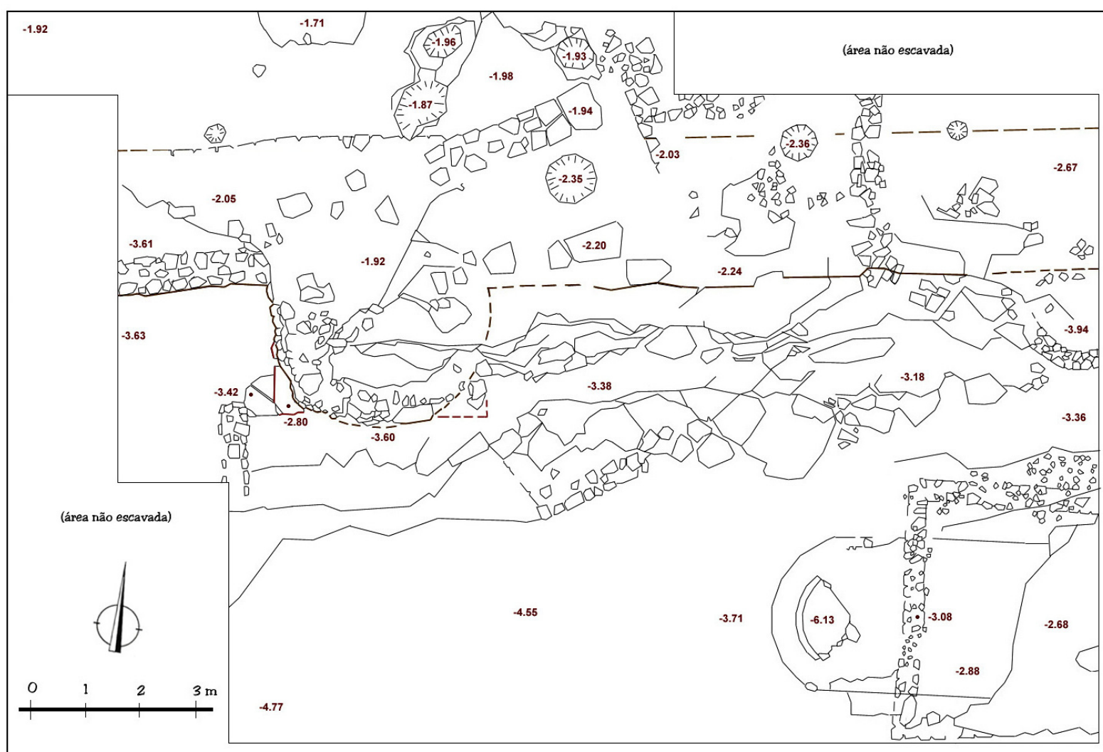
Planta da Sondagem F (des. Nuno Santos).
