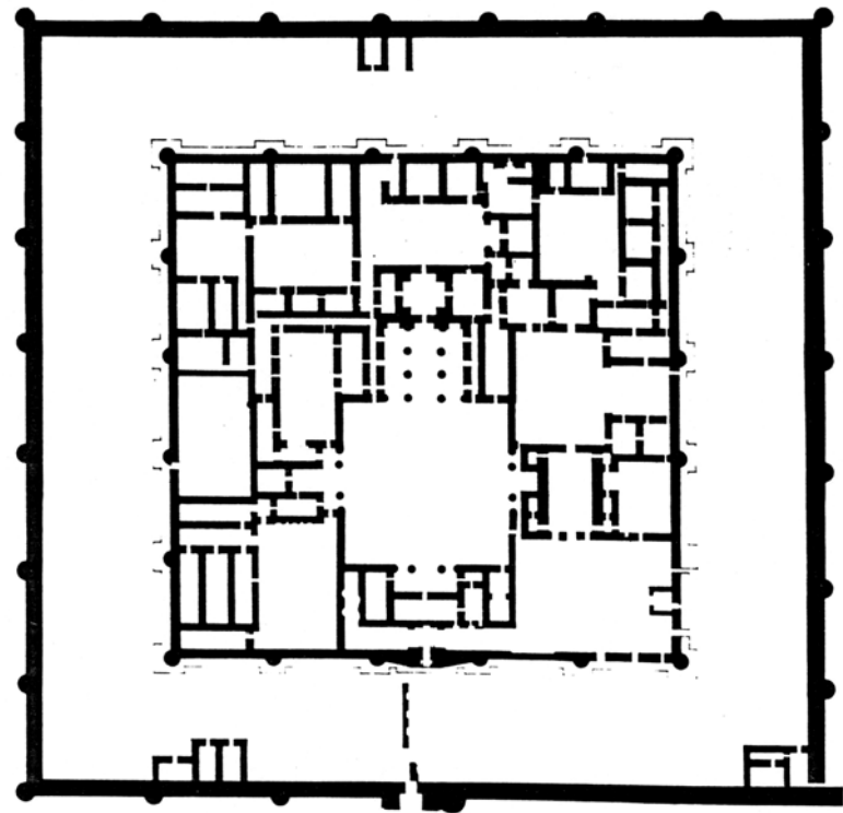
Planta do Palácio de Kufa (Iraque).
