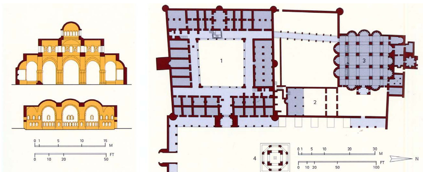
Khirbat al-Mafjar (Palestina).
