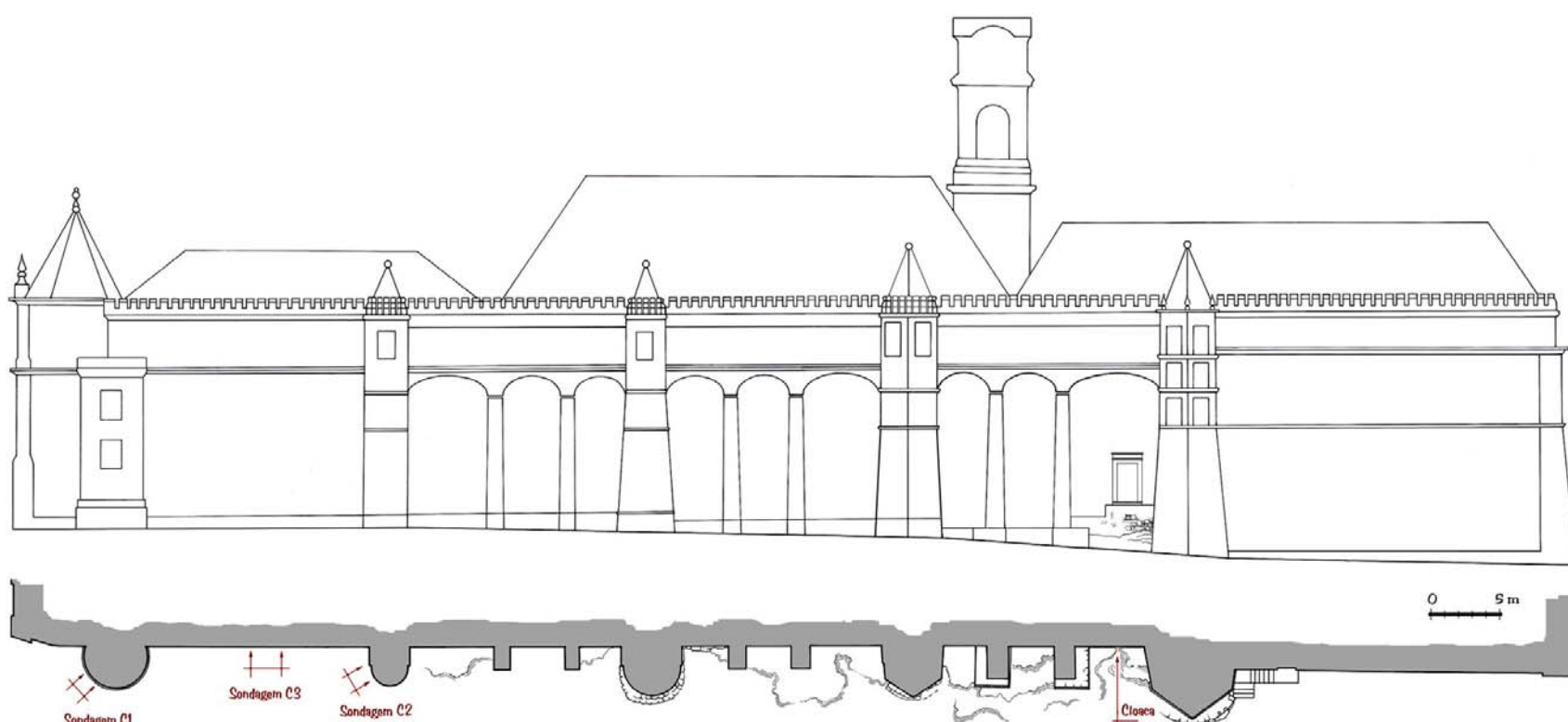
Alçado e planta da fachada norte (des. José Luís Madeira).
