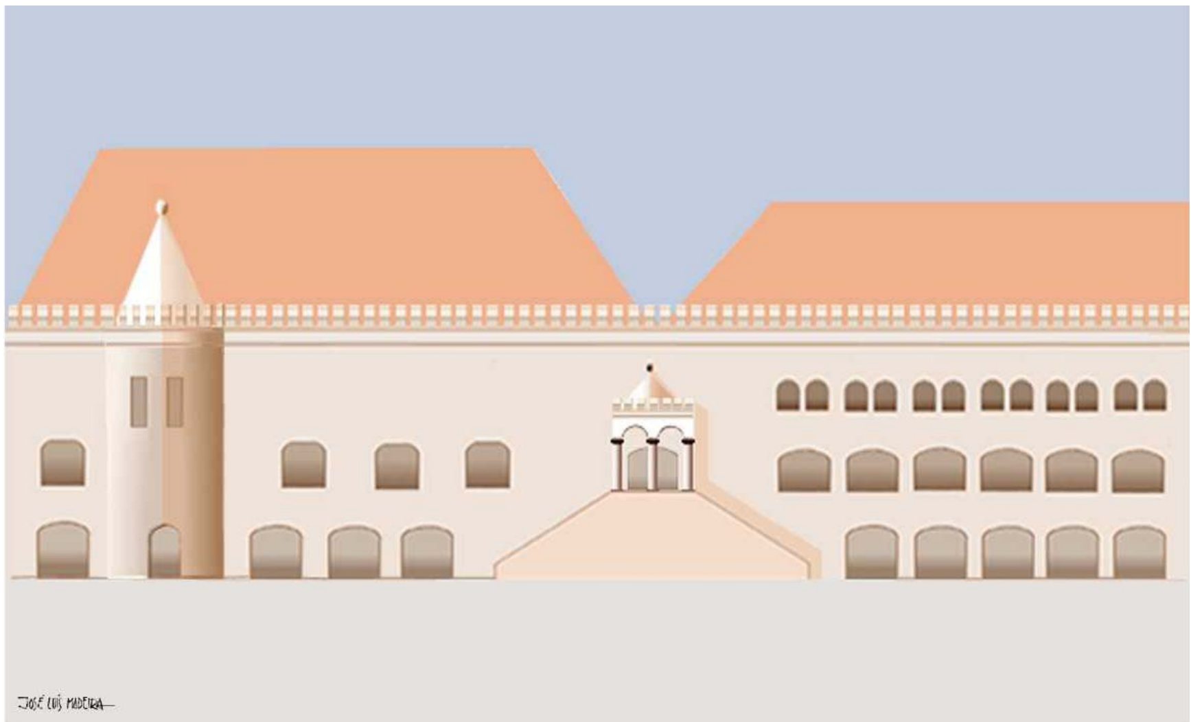
Reconstituição conjectural do alçado norte interno do Paço Real da Alcáçova, com a escadaria, eirado e coruchéu da Sala Grande e o cubelo voltado ao pátio (des. José Luís Madeira).
