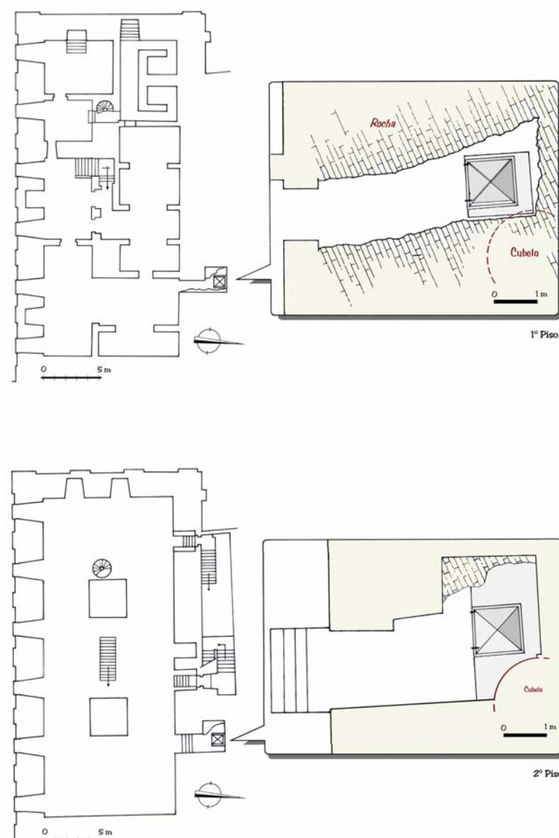
Implantação do cubelo de sudoeste (des. José Luís Madeira).
