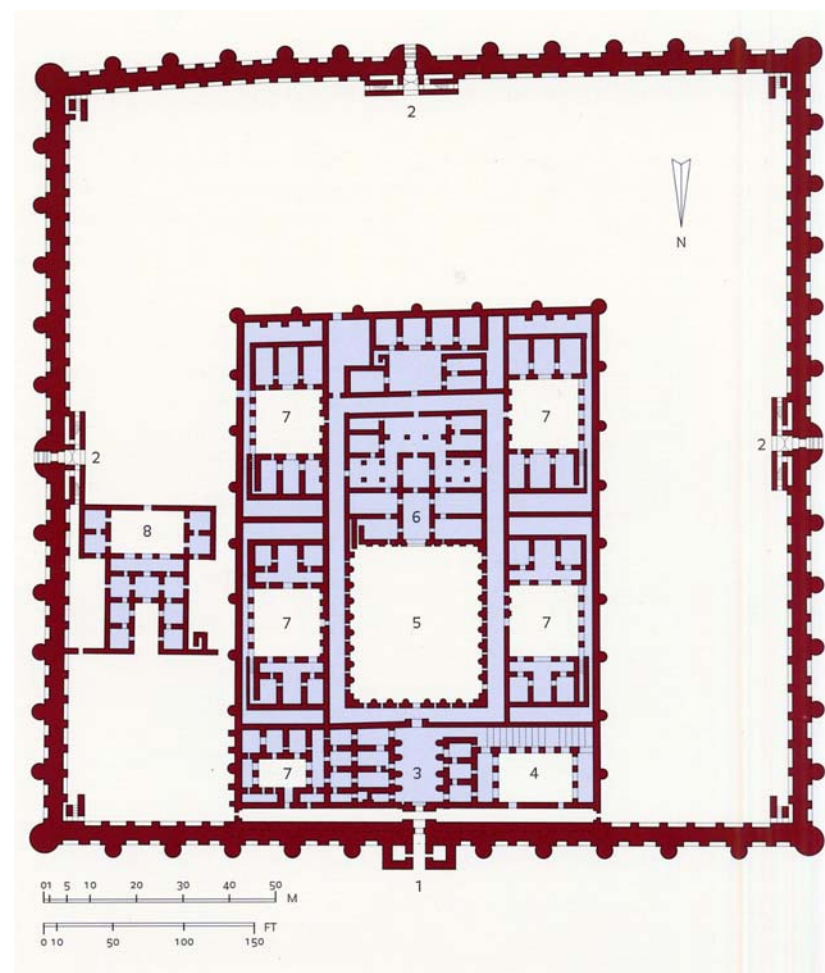
Planta do Palácio de Ukhaider (Iraque).
