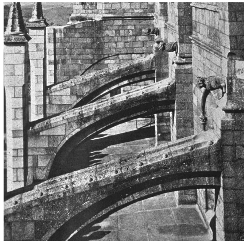
Aspecto da decoração perlada dos arcobotantes da Sé da Guarda.
