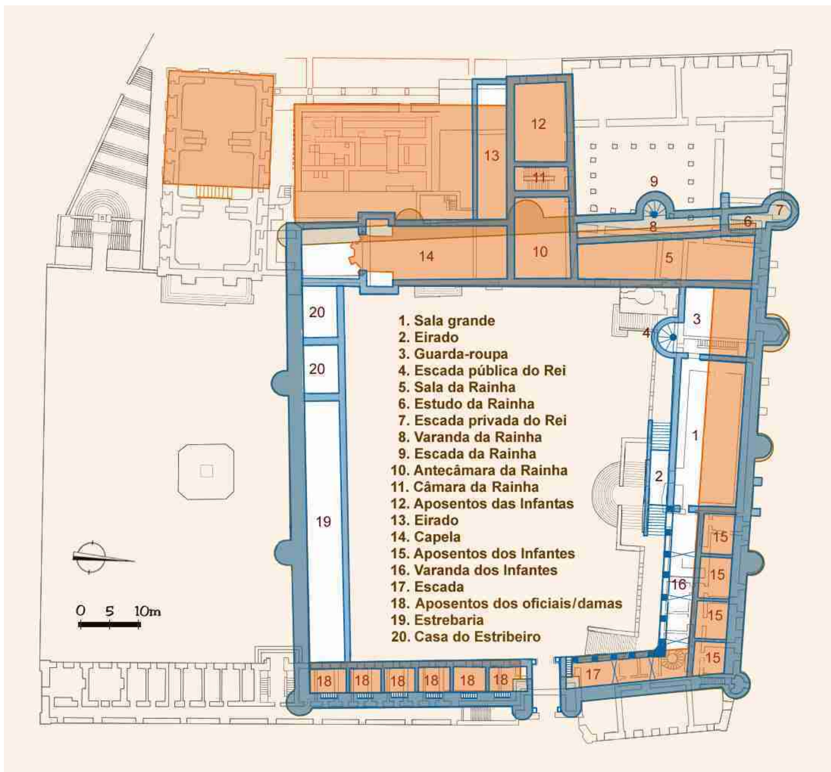
Reconstituição da distribuição do 1º piso (des. José Luís Madeira).
