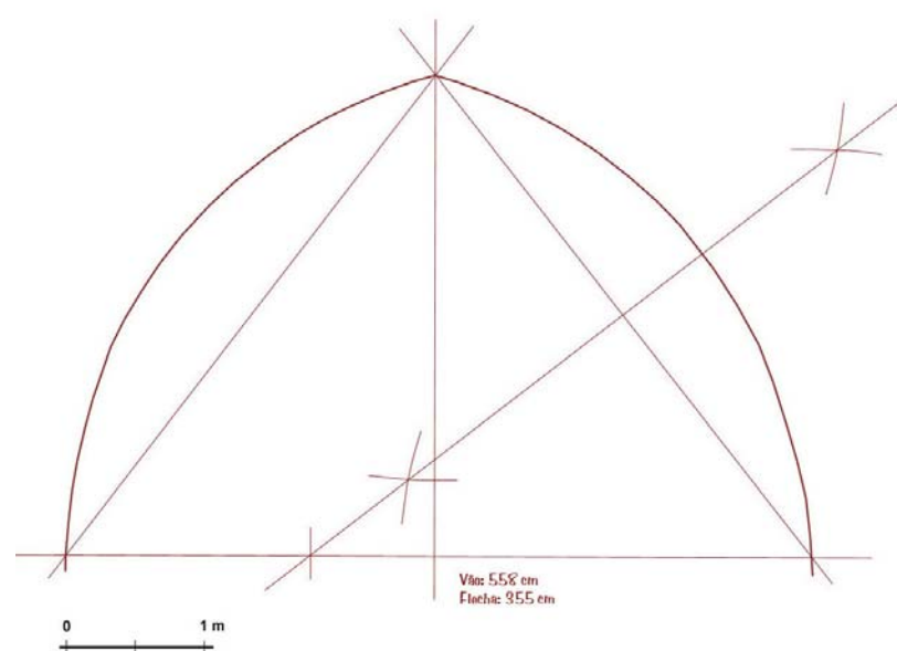
Reconstituição do traçado dos arcos quebrados (José Luís Madeira).
