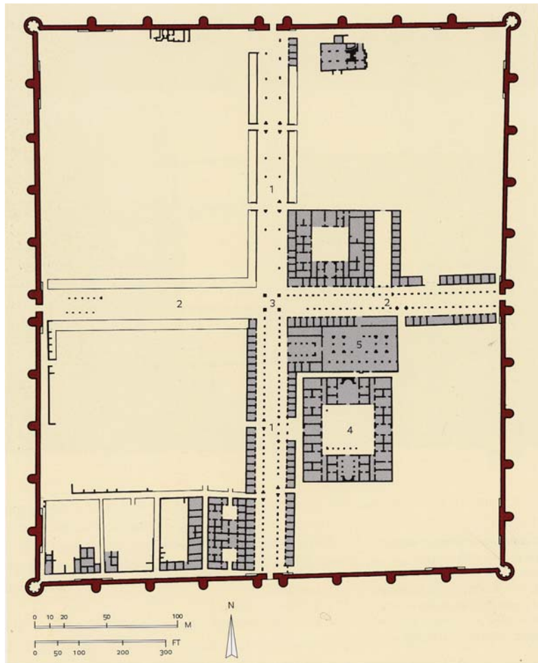
Planta do Palácio de Anjar (Líbano).
