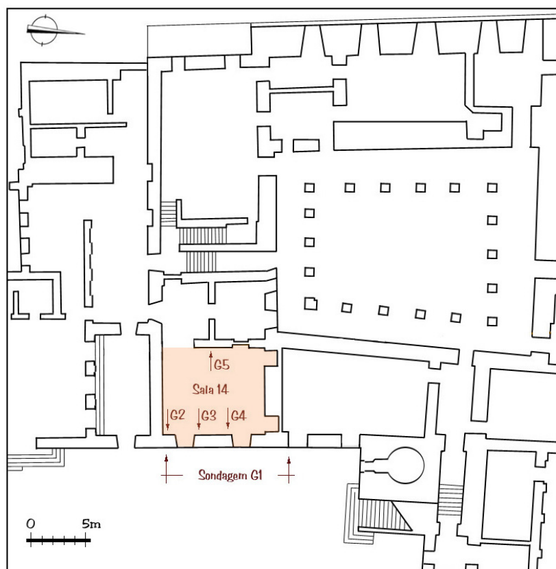
Localização das Sondagens G1, G2, G3, G4 e G5 (José Luís Madeira).
