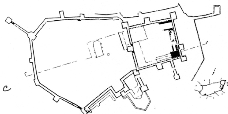
Planta do Castelo de Trujillo.
