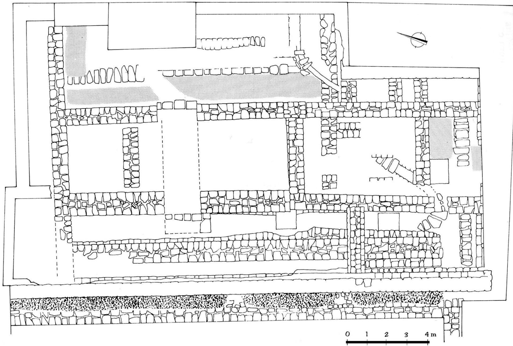
Intervenção arqueológica no Jardim da Capela (1979/81) (A. Nunes Pinto, Escavações na Alcáçova de Coimbra... ).
