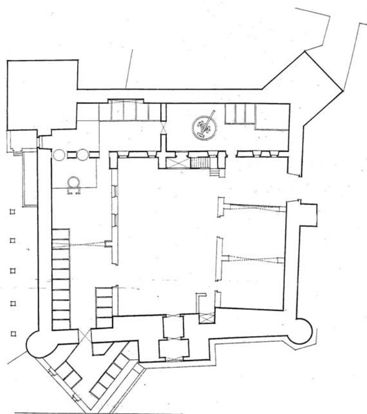
Planta do Castelo de Alter do Chão.
