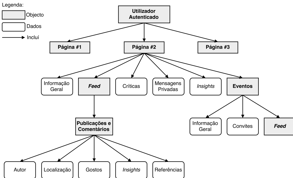
Figura 6.1: Estrutura dos dados extraídos do Facebook .
