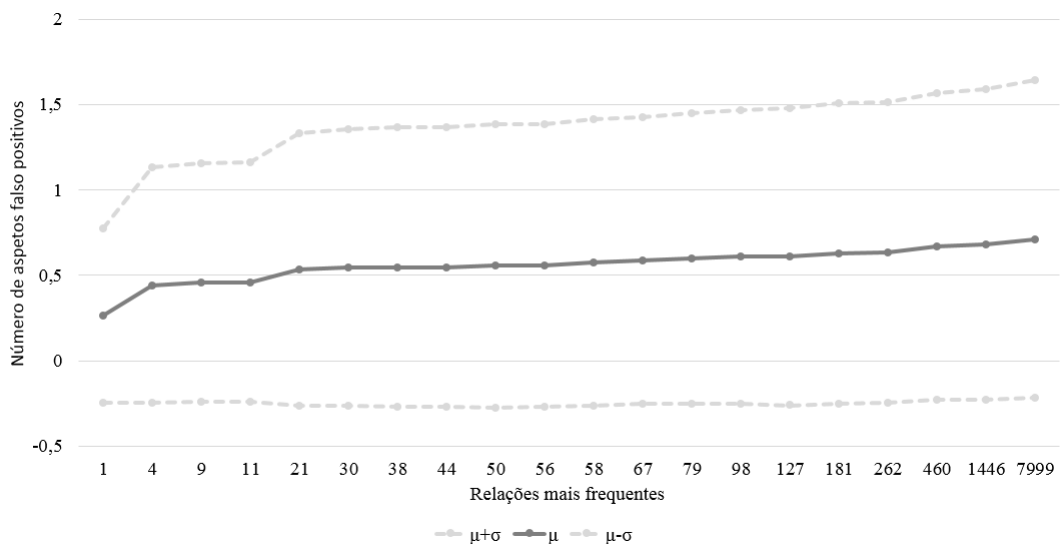
Figura 7.17: Média de número de aspetos falso positivos.
