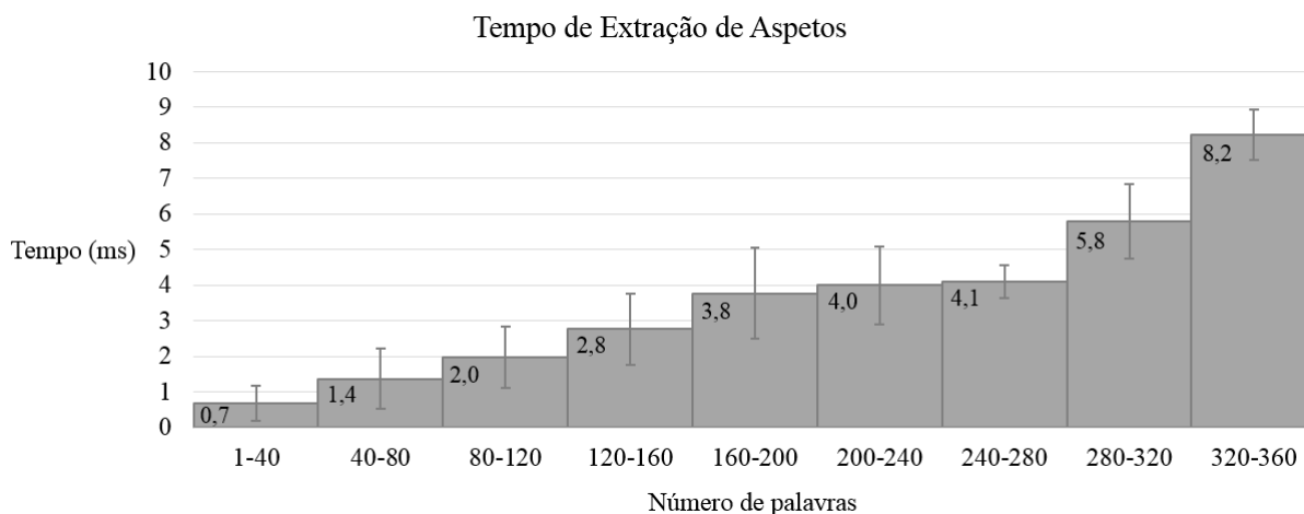
Figura 7.7: Tempo de extração de aspectos consoante o tamanho da frase.
