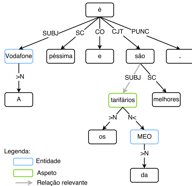
Figura 6.16: Exemplo de extração da relação entre entidades e aspetos para o Português.
