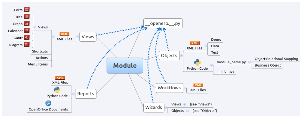
Figura 7.5: Estrutura de um Módulo no Odoo
